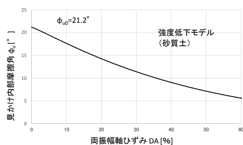
図5 標準強度低下モデル
