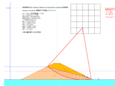
図6 臨界円弧の位置
