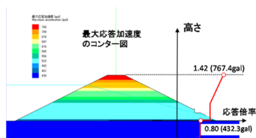
図3 堤体の応答加速度分布の例
