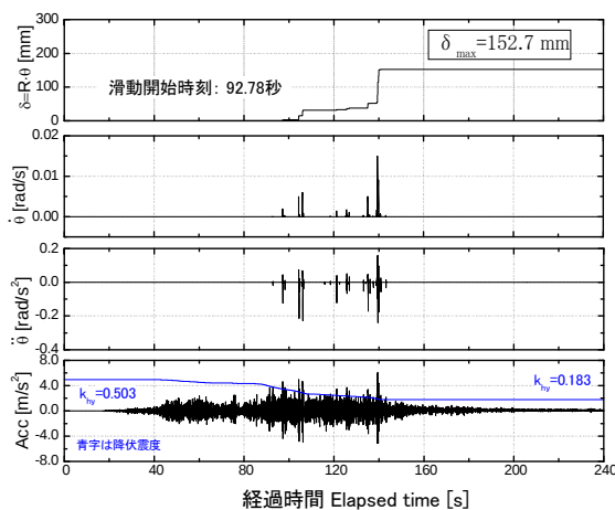
図7 滑動すべり量の計算結果
