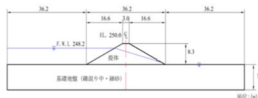
図4 解析断面
