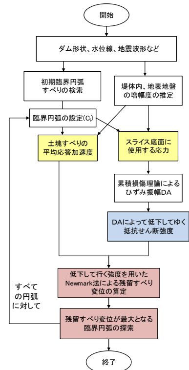
図 1 簡易 NewmarkD 法のフロー
