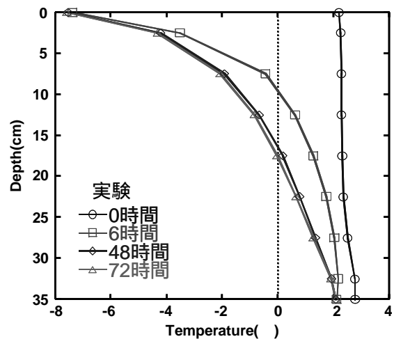
fig.2 温度分布
