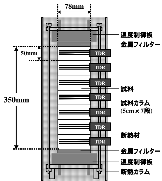
fig.1 凍結実験装置
