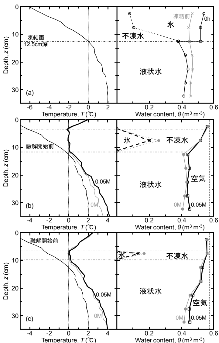
Fig. 1 融解開始後0, 24, 42hの温度・水分分布
