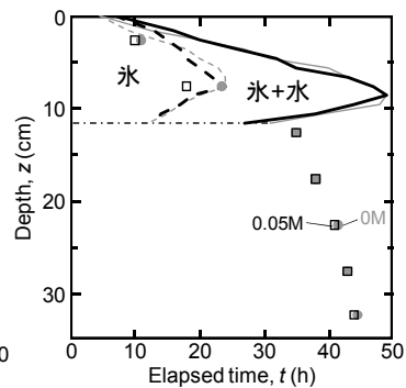
Fig. 3 浸潤前線と融解前線
