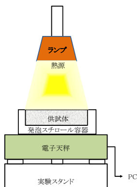
図1 実験装置の概略図
