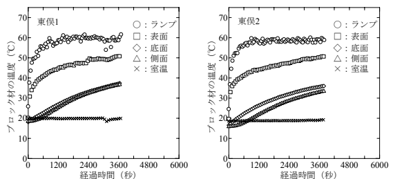
図3 ブロック材の温度変化（しらす50%）
