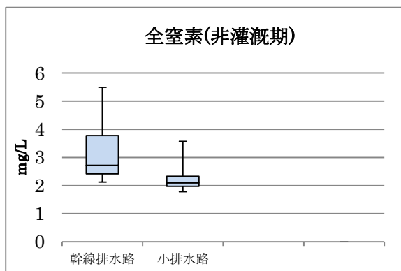
図3 非灌漑期の全窒素結果
