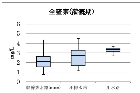
図2 灌漑期の全窒素結果
