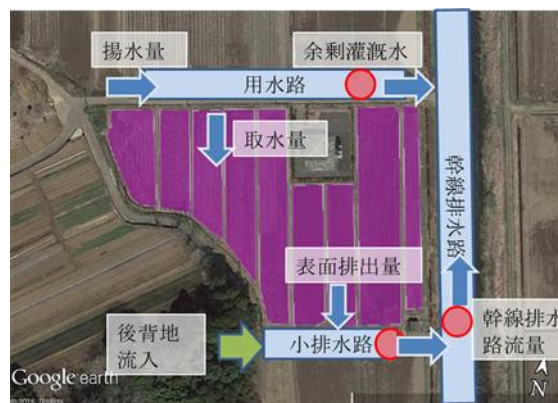
図1 調査地概要図
