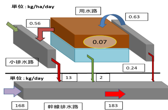
図4 灌漑期の全窒素収支
