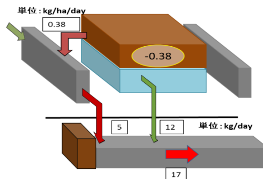
図5 非灌漑期の全窒素収支
